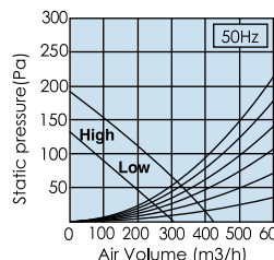
inWG (Pa) FV-38CH8
