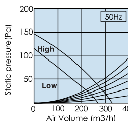
inWG (Pa) FV-38CD8
